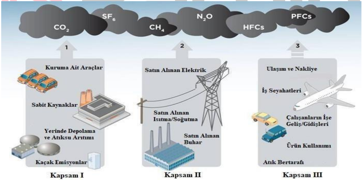
Şekil 3. Doğrudan ve Dolaylı Emisyonlar
