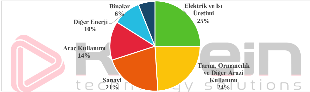
Şekil 2. Küresel Sera Gazları Emisyonlarının Ekonomik Sektörlere Göre Dağılımı 3
