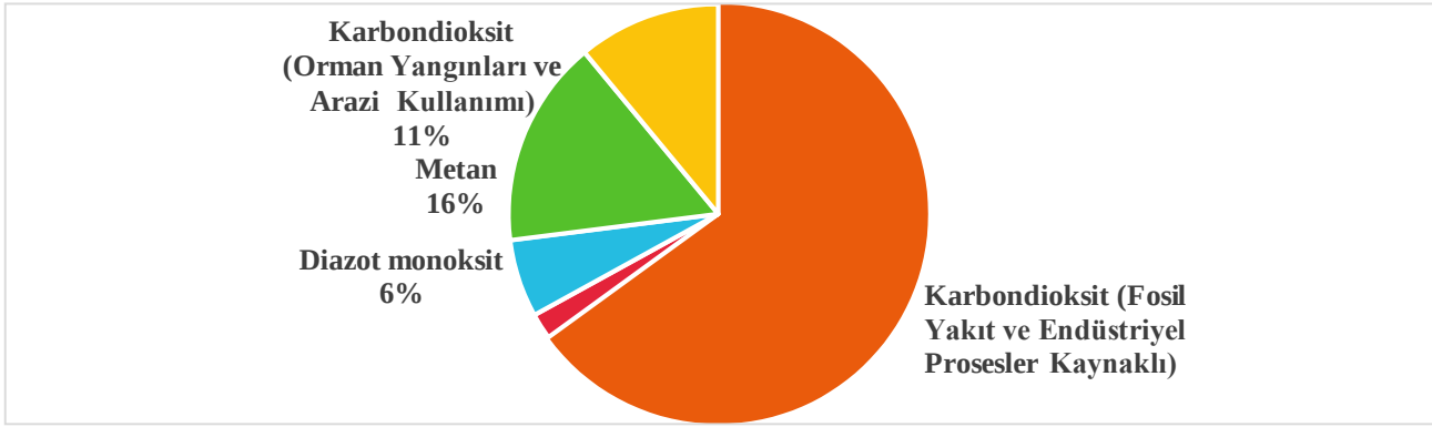
Şekil 1. Farklı Sera Gazlarının Küresel Isınmaya Etkileri2
